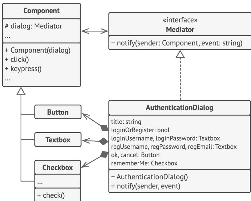
Estructura de las clases de diálogo UI.
