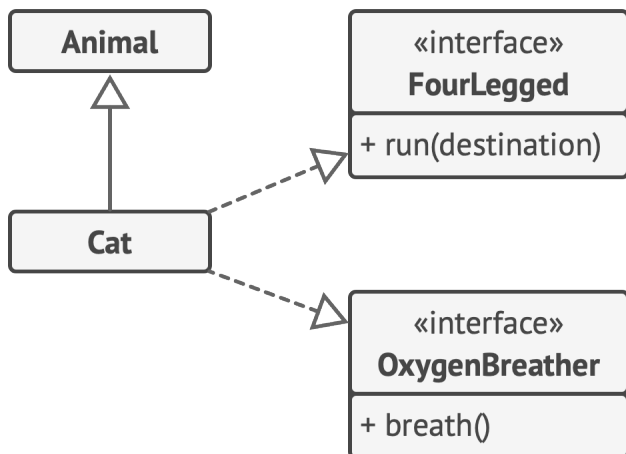
Diagrama UML de extensión de una única clase en comparación con la implementación de múltiples interfaces al mismo tiempo.
