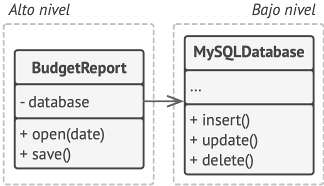
ANTES: una clase de alto nivel depende de una clase de bajo nivel.
