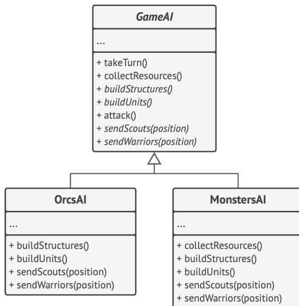
Clases IA de un sencillo videojuego.
