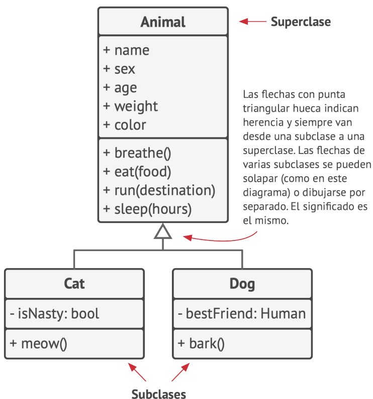
Diagrama UML de una jerarquía de clases. Todas las clases de este diagrama son parte de la jerarquía de clases Animal .
