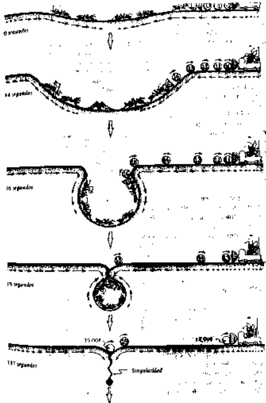
Fig. 1.1] colapso de una membrana elástica poblada por bolitas proporcionala una final- 164 lica analoga de la implosión gravitatoria de una estrella para formar un agujero ne- 165 tro. [Adaptado de Thorne (1967).]
