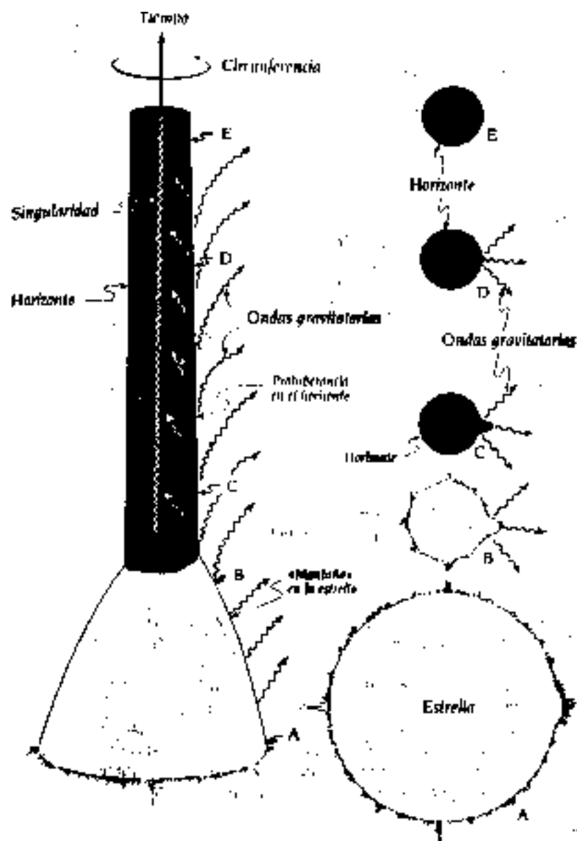
7.4. Diagrama espacio-temporal ( izquierda ) y una secuencia de instantáneos ( derecha ) que muestran la implosión de una estrella con una montaña para formar un agujero negro.
