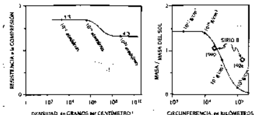
4.3. Esquema de la ecuación de estado de Shönner-Anderson para la materia de las enanas blancas, es decir, la relación entre la densidad de la materia y su resistencia a la compresión. En horizontal se representa la densidad a la que ha sido comprimida la materia. En vertical se representa su resistencia (el incremento porcentual de presión que acompaña a un 1 por 100 de incremento de densidad). A lo largo de la curva se ha marcado la presión de compresión (igual a la presión interna), en múltiplos de la presión atmosférica. Derecha: las circunferencias (representadas en horizontal) y masas (representadas en vertical) de estrellas enanas blancas calculadas por Chandrasekhar utilizando la calculadora mecánica Braunschweiger de Eddington. A lo largo de la curva se ha marcado la densidad de la materia en el centro de la estrella, en gramos por centímetro cúbico. 3
