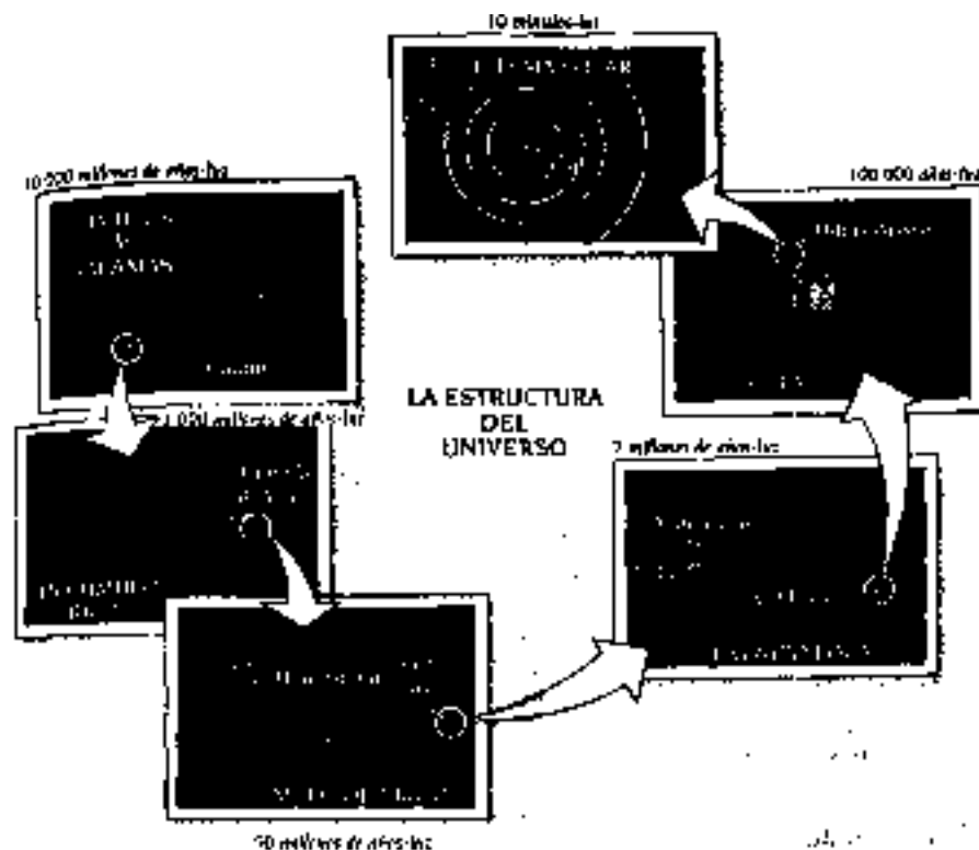
R.1. Un esbozo de la estructura de nuestro Universo.
