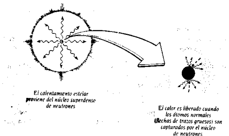
5.4. Especulación de Lev Landau sobre el origen de la energía que mantiene caliente una estrella normal.
