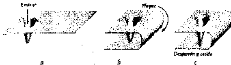
14.4. Una estrategia para hacer un agujero de gusano: a) Se crea un «calceón» en la curvatura del espacio. b) El espacio fuera del calceón se dobla suavemente en el hiperespacio. c) Se rasga un pequeño agujero en el fondo del calceón, se rasga un agujero en el espacio justo debajo del agujero, y se «cosen» los bordes de los agujeros. Esta estrategia parece clásica (macroscópica) a primera vista. Sin embargo, el rasgado produce, al menos momentáneamente, una singularidad espacio-temporal que está gobernada por las leyes de la gravedad cuántica, de modo que esta estrategia es realmente cuántica.
